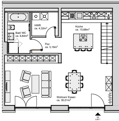
ERDGESCHOSS
